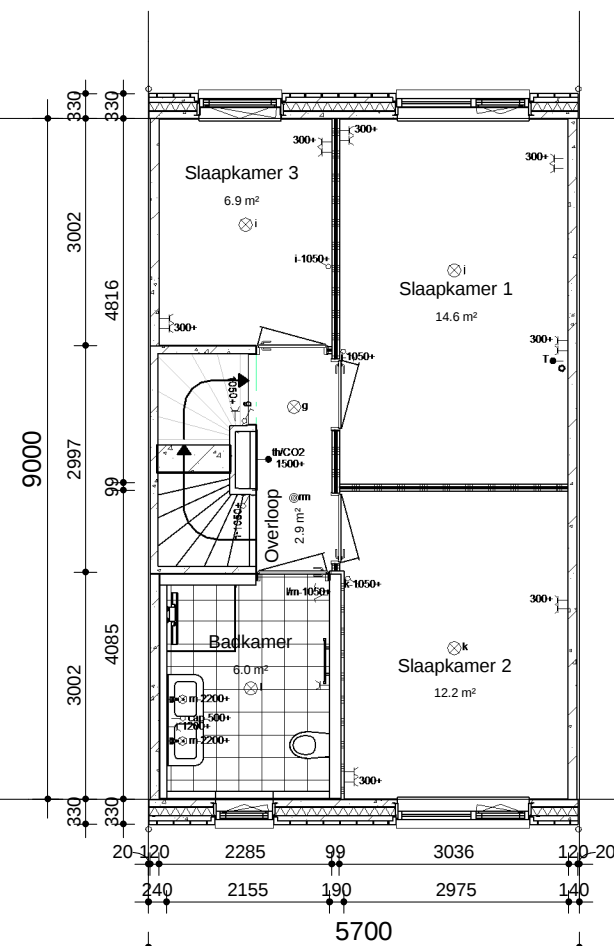
1e VERDIEPING
