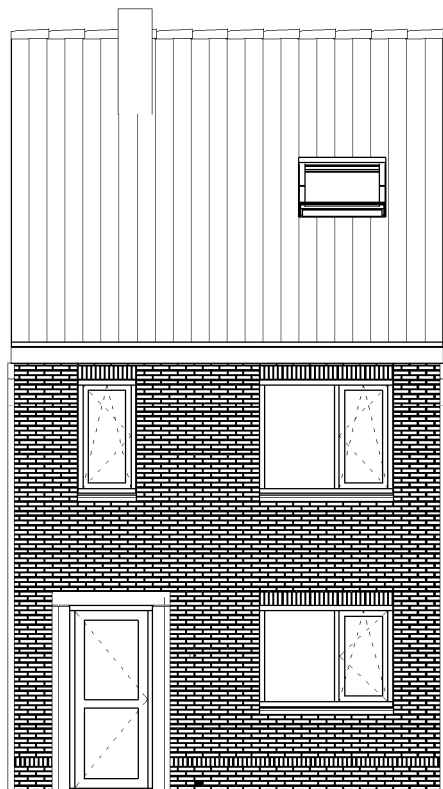
VOORGEVEL
