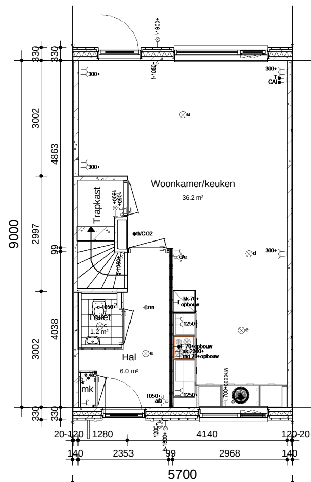
BEGANE GROND
