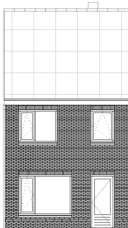
ACHTERGEVEL
